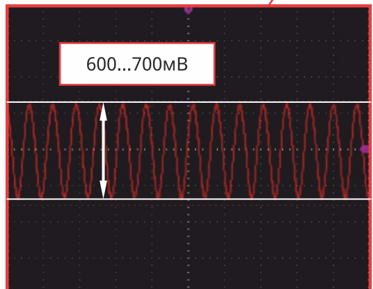
Контрольная точка TP1
