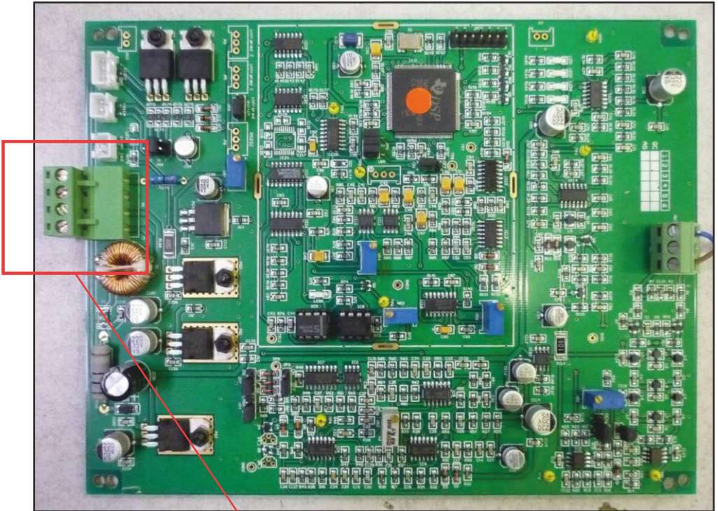
Разъёмы питания
